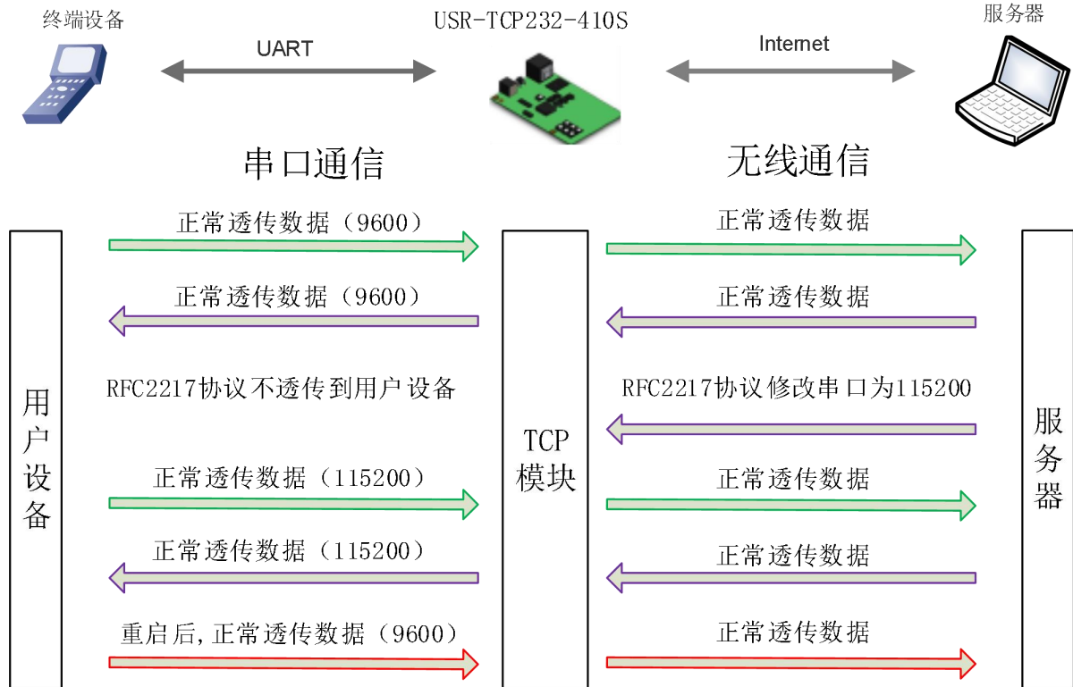
图 24 类 RFC2217 功能框图
