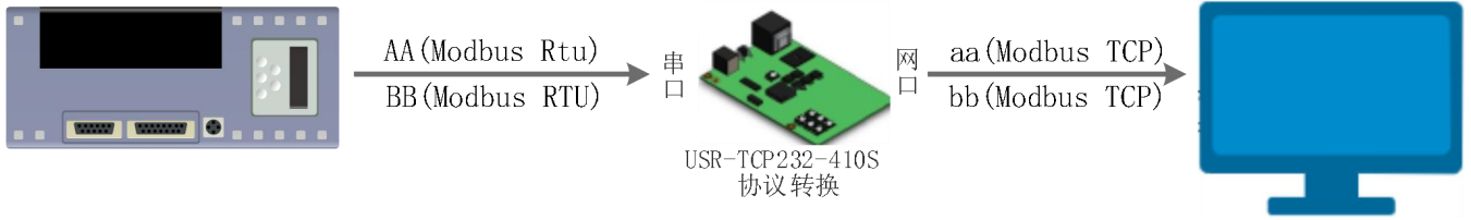
图 28 Modbus TCP
