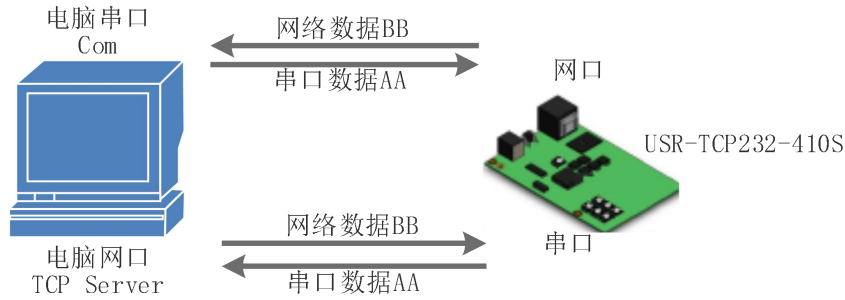
图 2 数据流向
