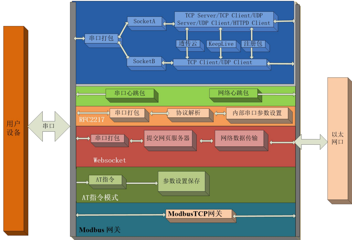
图 7 410s 功能框图
