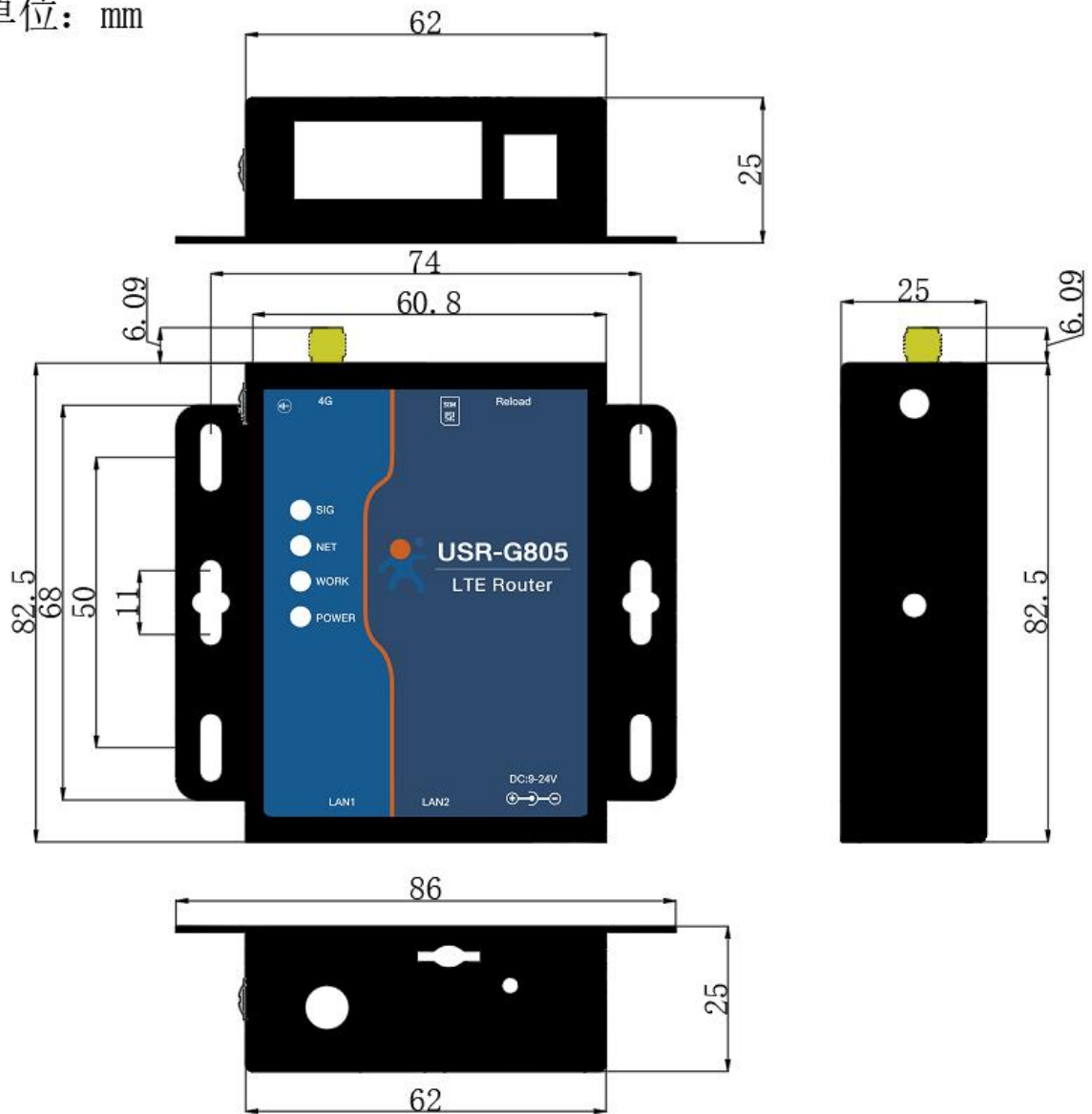
USR-G805 产品尺寸
